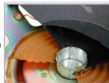
La coupe dans le moteur du haut-parleur : bobine et suspension.
